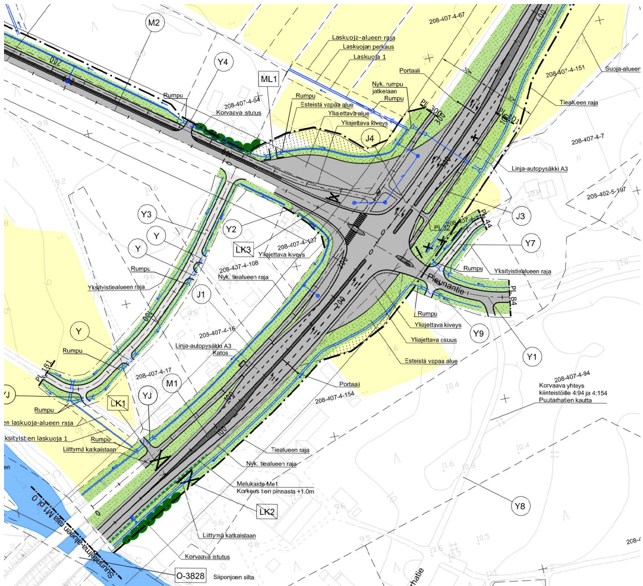
Kuva 9: Karttaote Kalajoen vt 8 / yt 7771-liittymän (POS A1) risteysalueen järjestelyiden parantamisen suunnitelmakartan luonnoksesta. Suunnitelma oli ELY-keskuksessa esitarkastuksessa 30.9.2024.
