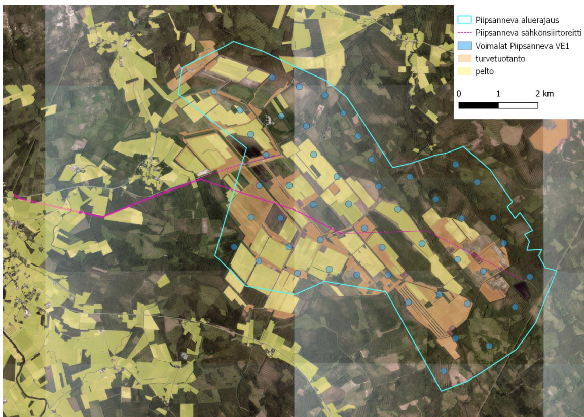
Kuva 8. Voimaloiden sijoittuminen hankevaihtoehdossa VE1
